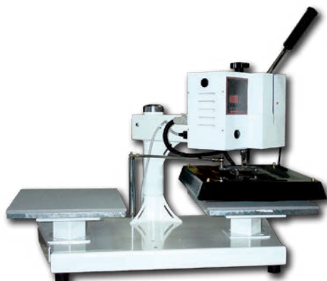
Pressa manuale ad apertura laterale con due piatti cm 35 x 45
