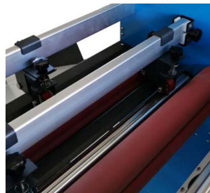
Separatore carta
